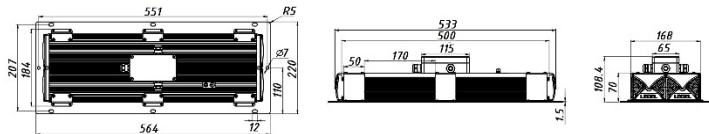
Рисунок 1 Общий вид светильника «L-industry NEW 48 A3C»
